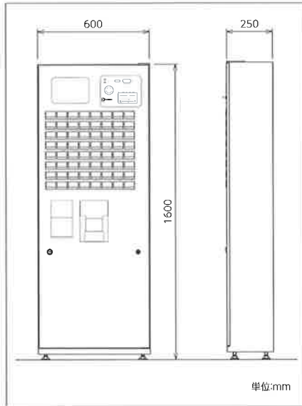
寸法図
